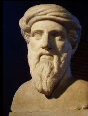
Пифагор
