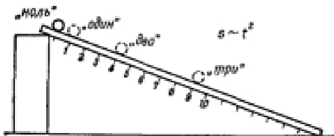
Рисунок 3.2. Опыт Галилея.
